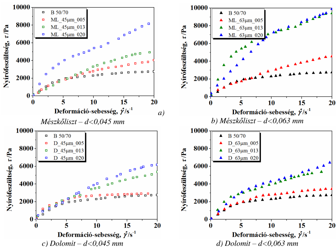
6. ábra. Aszfalthabarcok összesített valódi folyásgörbéi ( T=60^\circ C )
